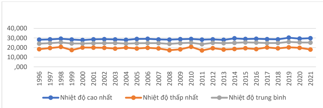
Hình 1. Biến động nhiệt độ không khí ở tỉnh Thừa Thiên Huế, giai đoạn 1996- 2021
