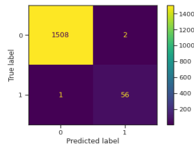
Hình 10. Hiệu suất của mô hình Random Forest
