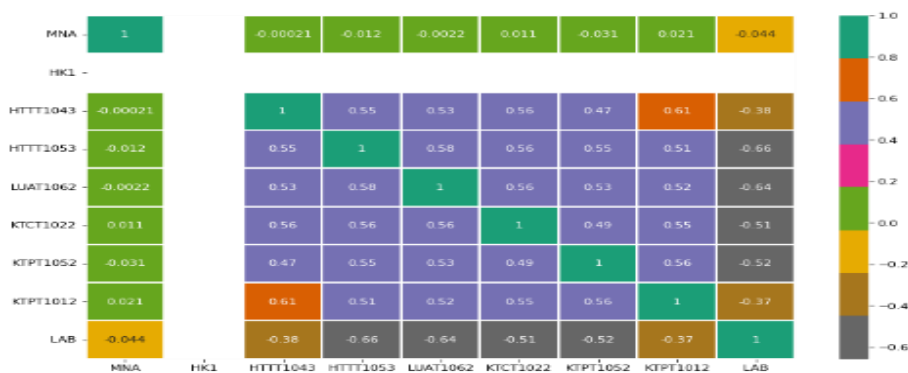
Hình 4: Tương quan dữ liệu
