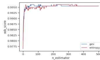
Hình 9. Biểu đồ Oob_score
