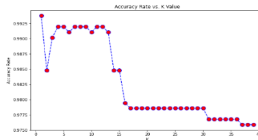
Hình 8: Tìm k tối ưu trong mô hình kNN
